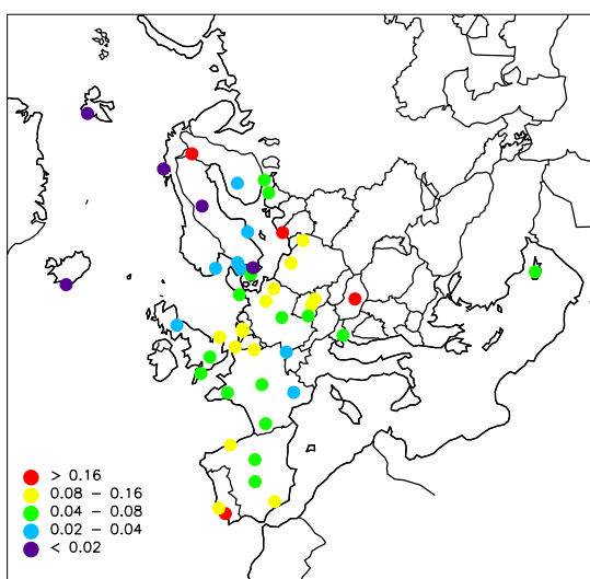
Fig. 1.5. Cd in aerosol, ng/m 3
